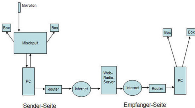
Radio Intertape Live Vereinfachte, schematische Darstellung
